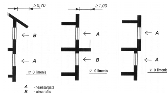
Logu vai durvju klasifikācija ūdens necaurlaidības noteikšanai
